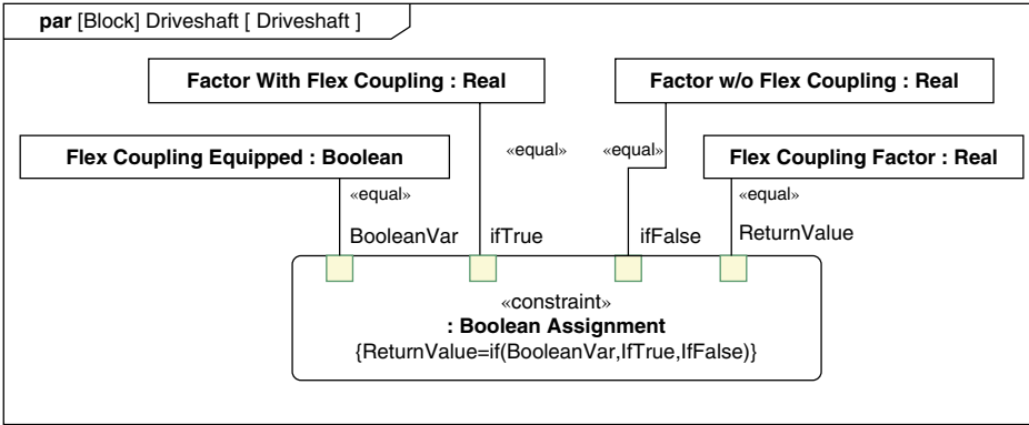
Figure 10.8. SysML parametric diagram.
