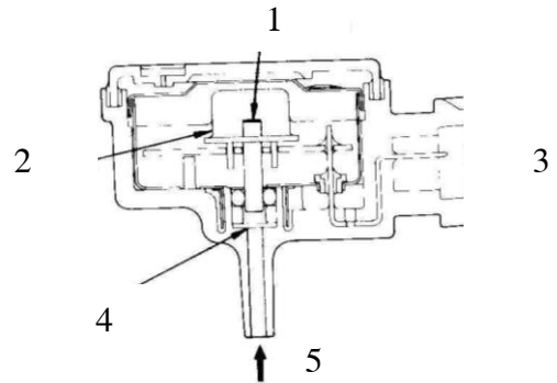
Hình 24: Cảm biến áp suất đường ống nạp
