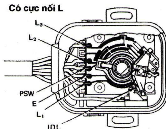
Hình 46: Cảm biến cánh bướm ga có thêm vị trí tay số
