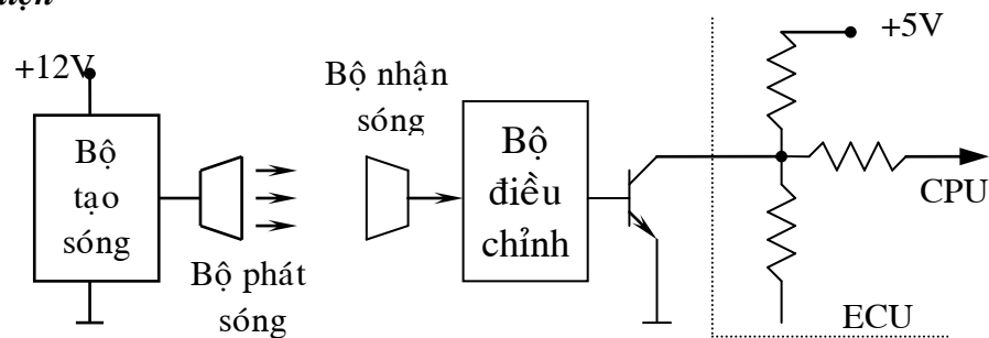
Hình 20: Mạch điện cảm biến đo gió Karman siêu âm
