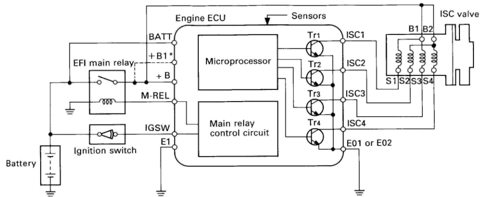
Hình 149: Mạch điện của kiểu motor bước
