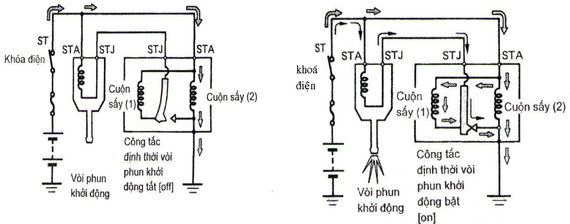
Hình 138: Mạch điện công tắc nhiệt thời gian
