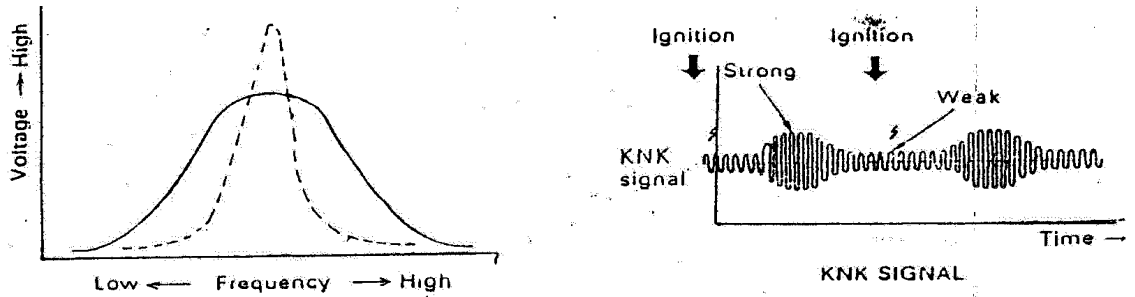
Hình 63: Đồ thị biểu diễn tần số kích nổ
