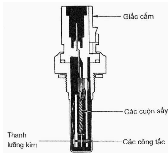
Hình 137: Công tắc nhiệt thời gian
