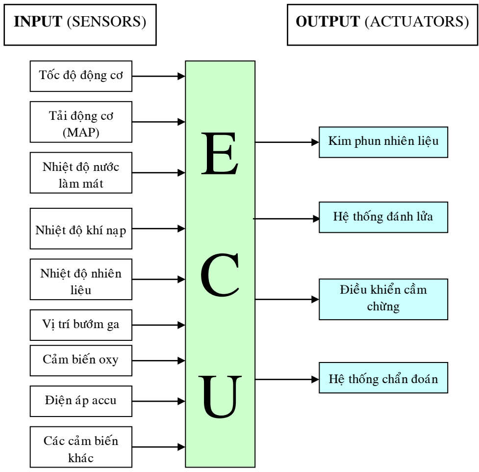
Hình 2: Sơ đồ cấu trúc của hệ thống điều khiển lập trình cho động cơ
