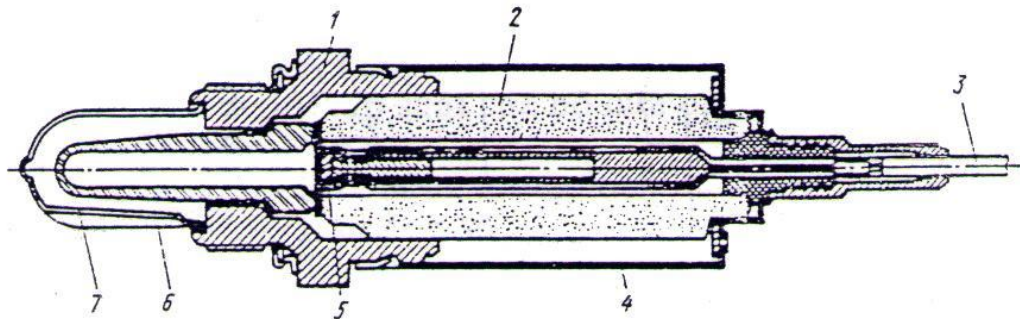
Hình 56: Cấu tạo cảm biến oxy loại Zirconium
