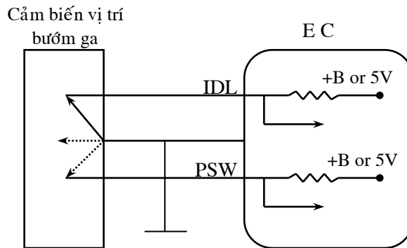
Hình 42: Mạch điện cảm biến vị trí cánh bướm ga loại âm chờ
