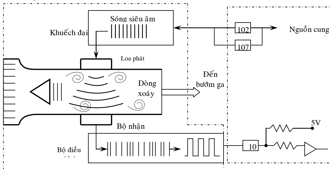
Hình 14: Cấu trúc cảm biến đo gió Karman kiểu siêu âm
