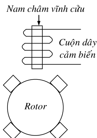
Hình 31: Sơ đồ nguyên lý của loại dùng cảm biến điện từ
