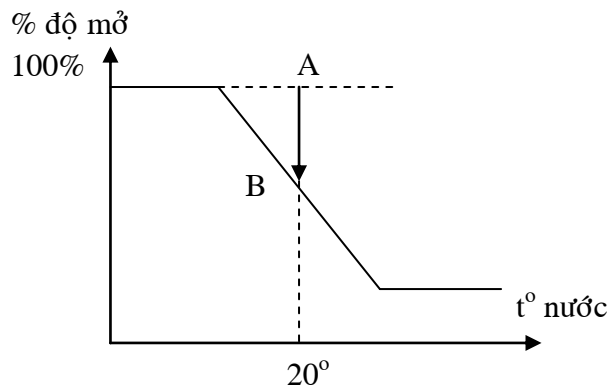
Hình 142: Điều khiển cầm chừng ở chế độ sau khởi động
