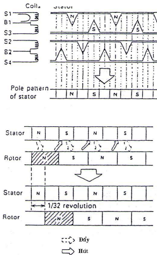
Hình 148: Hoạt động của motor bước
