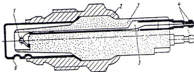
Hình 58: Cảm biến oxy loại titanium
