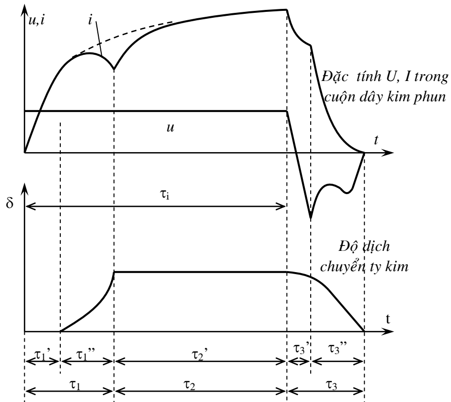
Hình 121: Đặc tính u, i, \delta = f(t) trong cuộn dây kim phun
