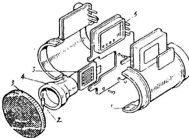
Hình 23: Cảm biến đo gió loại màng nhiệt
