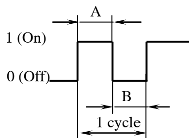
Hình 151: Dạng xung của kiểu Solenoid
