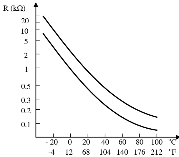
Hình 52: Đường đặc tuyến của cảm biến nước làm mát
