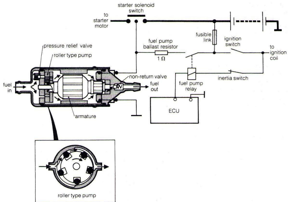
Hình 111: Bơm con lăn
