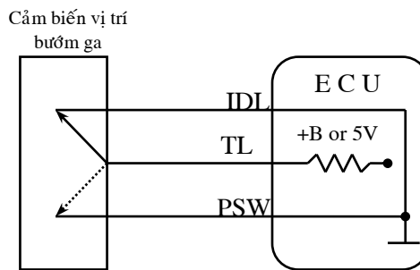
Hình 43: Mạch điện cảm biến vị trí bướm ga loại dương chờ
