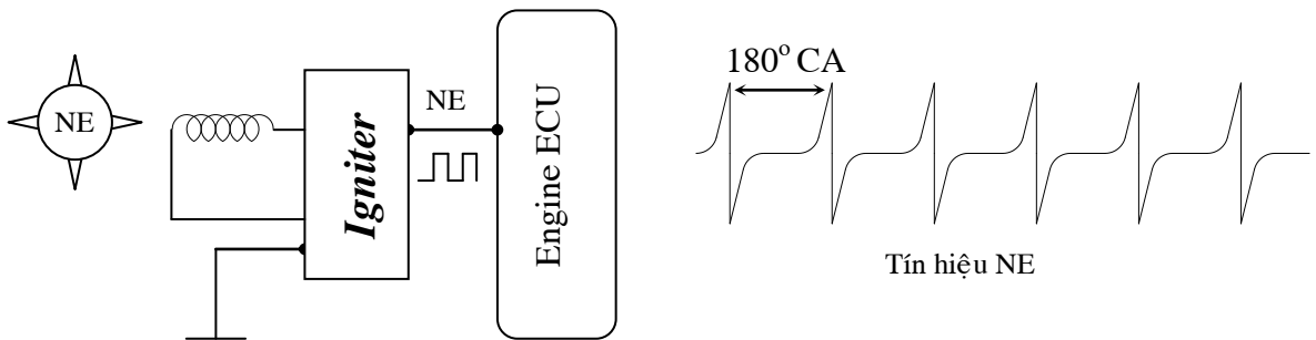
Hình 35: Sơ đồ và dạng xung loại 1 cuộn dây chung cho G và NE kết hợp với IC đánh lửa
