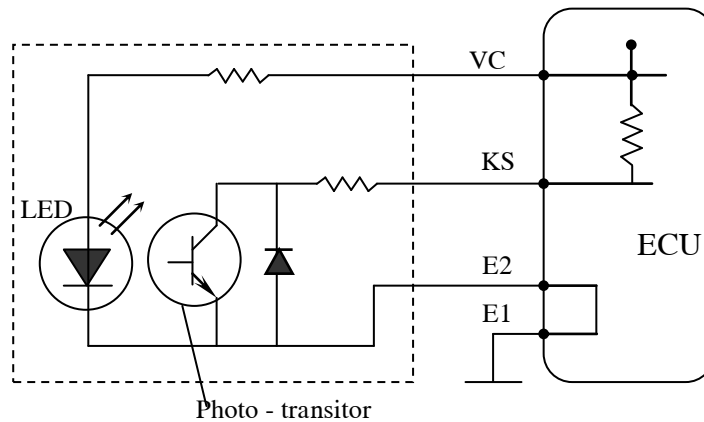
Hình 13: Mạch điện đo gió kiểu Karman quang
