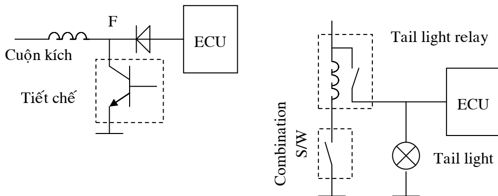
Hình 145: Điều khiển cầm chừng theo tải máy phát
