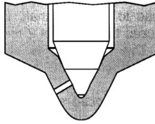
Hình 7.11: Cấu tạo đầu kim lỗ tia hở
