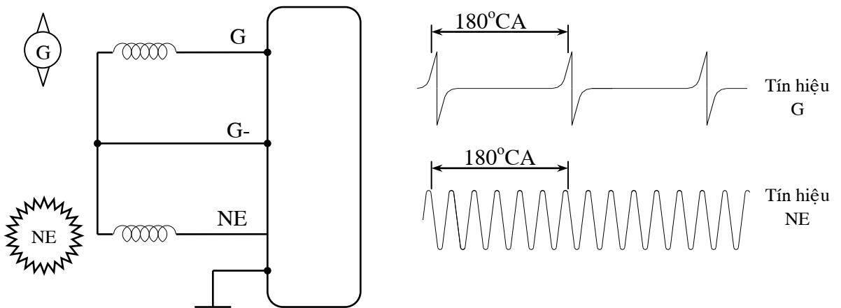
Hình 33: Sơ đồ và dạng xung loại 2/24
