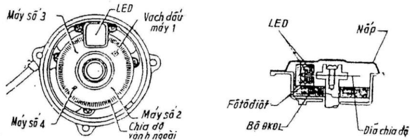
Hình 39: Cấu tạo cảm biến quang
