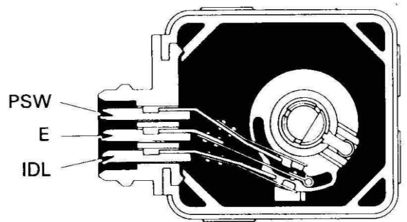
Hình 41: Cảm biến cánh bướm ga loại công tắc
