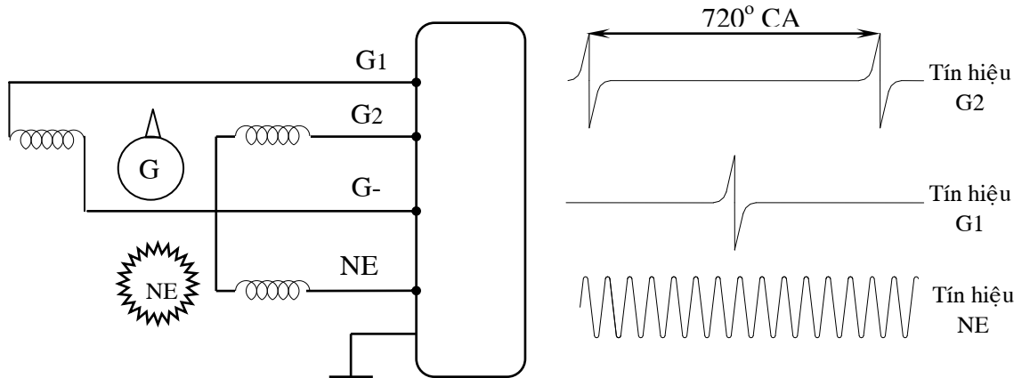
Hình 34: Sơ đồ và dạng xung loại 1/24
