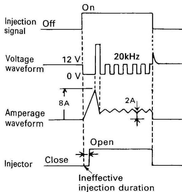
Hình 126: Phương pháp điều khiển kim phun bằng dòng
