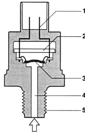
Hình 7.12: Cảm biến áp suất trên ống phân phối
