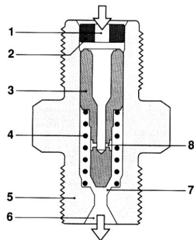
Hình 7.14: Van giới hạn dòng chảy
