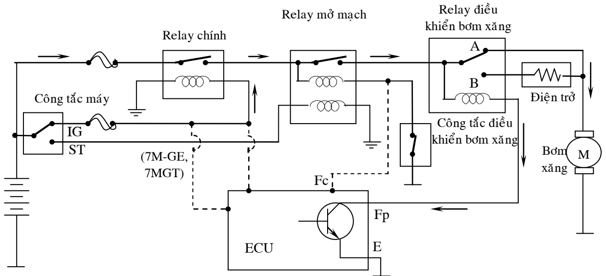
Hình 115b: Mạch điện điều khiển bơm xăng qua ECU điều khiển tốc độ bơm
