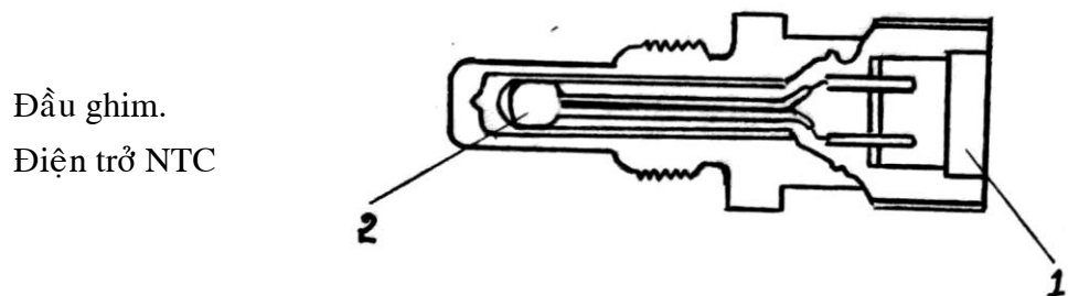
Hình 53: Cảm biến nhiệt độ khí nạp
