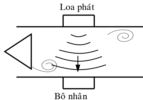
Hình 18: Dòng khí ngược chiều sóng siêu âm
