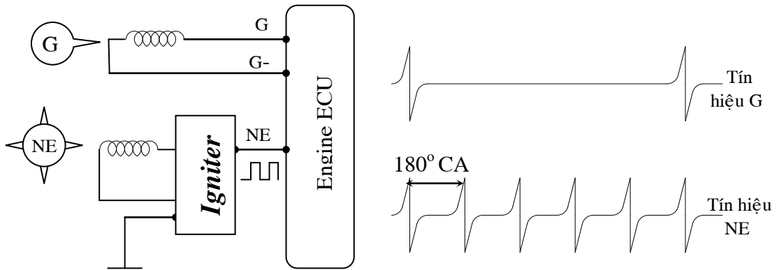
Hình 32: Sơ đồ mạch điện và dạng tín hiệu xung G và NE.
