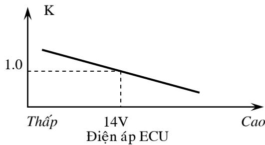
Hình 136: Hiệu chỉnh lượng phun theo điện áp
