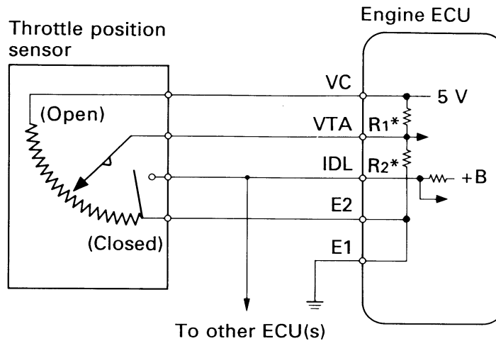
Hình 45: Mạch điện cảm biến vị trí cánh bướm ga loại biến trở
