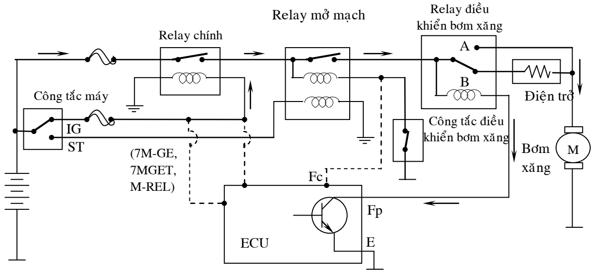
Hình 115a: Sơ đồ điều khiển bơm xăng qua ECU với mạch điều khiển tốc độ
