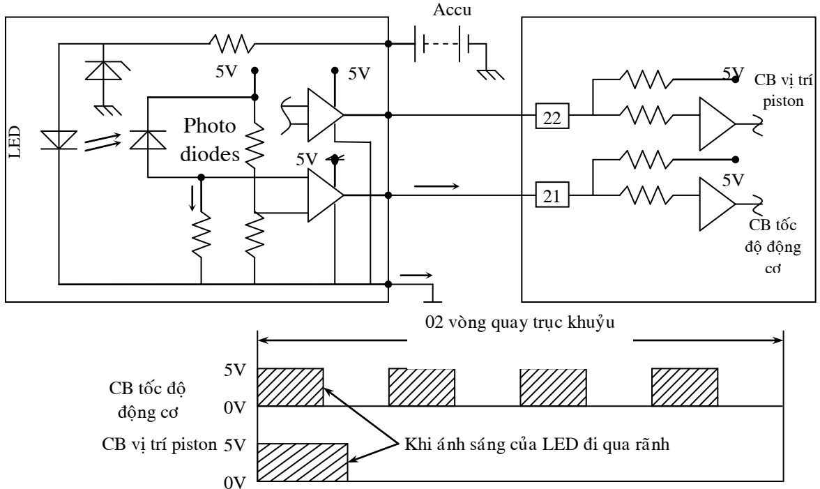
Hình 40: Mạch điện cảm biến quang và dạng xung ra
