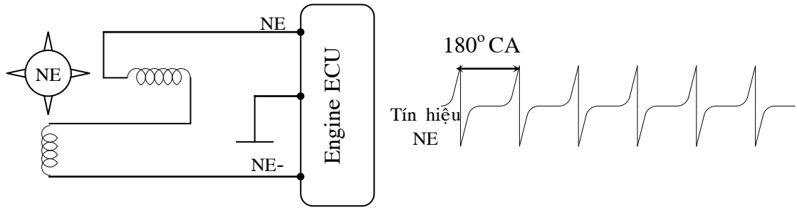
Hình 37: Sơ đồ và dạng xung loại 2 cuộn dây chung cho G và NE
