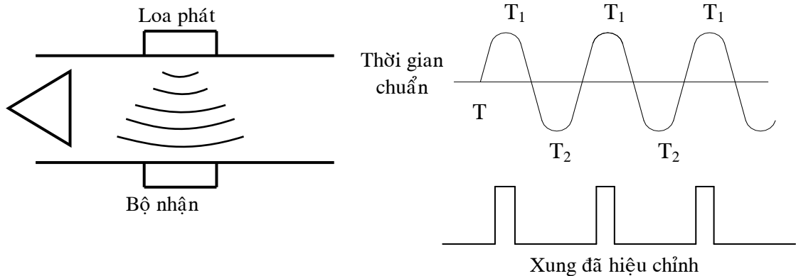
Hình 16: Bộ phát sóng và dạng xung
