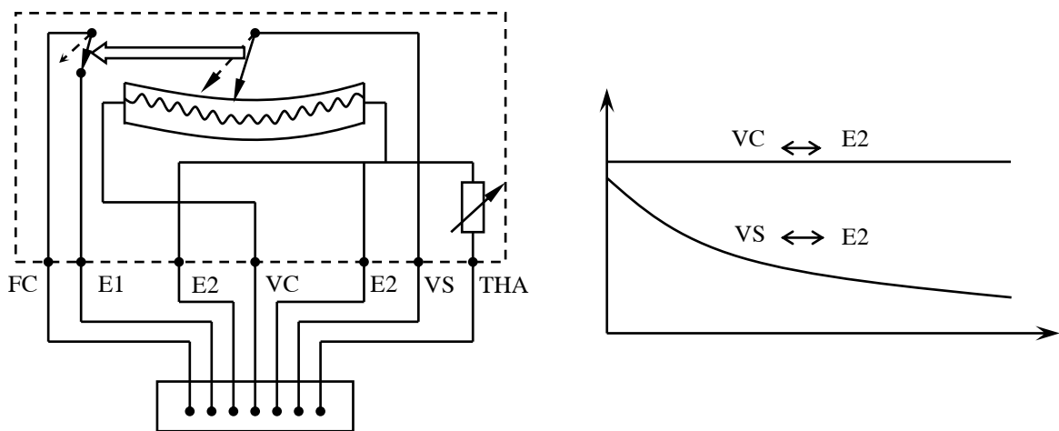
Hình 10: Mạch điện và đường đặc tuyến cảm biến đo gió loại điện áp giảm
