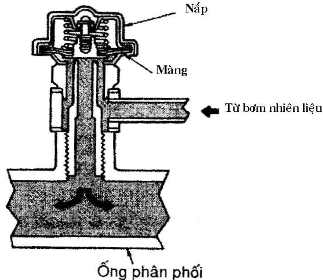
Hình 116: Bộ giảm dao động
