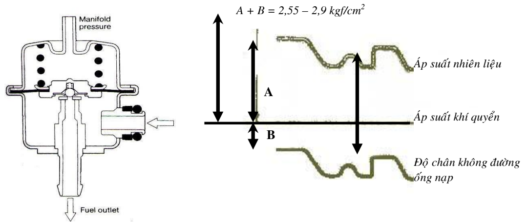
Hình 117: Bộ điều áp và đặc tính hoạt động
