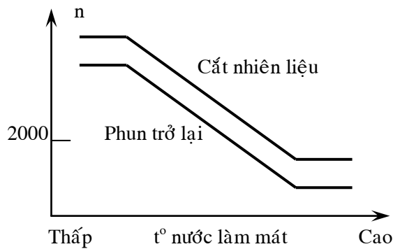
Hình 135: Đồ thị biểu diễn sự cắt nhiên liệu
