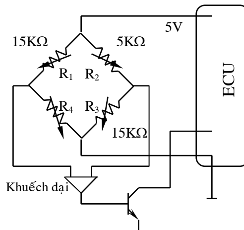
Hình 25: Sơ đồ nguyên lý cảm biến áp suất đường ống nạp
