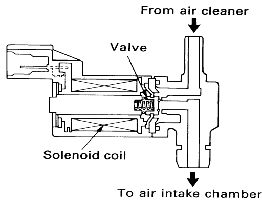
Hình 150: Cấu tạo của kiểu solenoid
