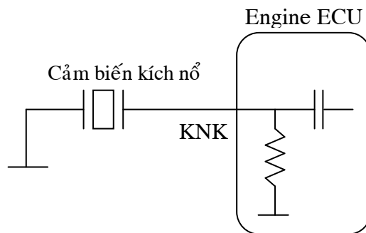
Hình 64: Mạch điện cảm biến kích nổ
