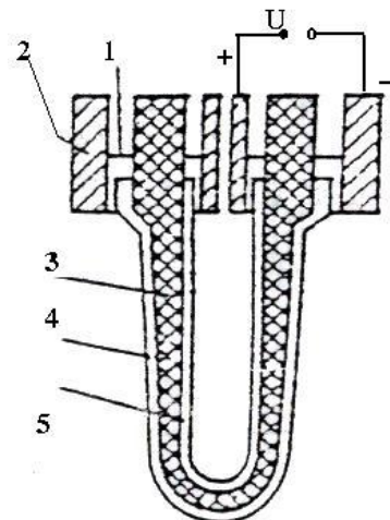
Hình 55: Cảm biến với thành phần zirconium
