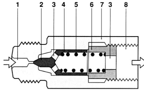
Hình 7.13: Van giới hạn áp suất
