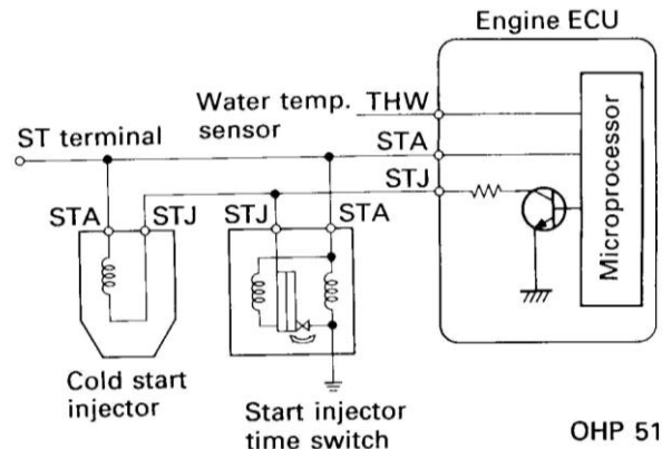
Hình 140: Mạch điện kim phun khởi động lạnh
