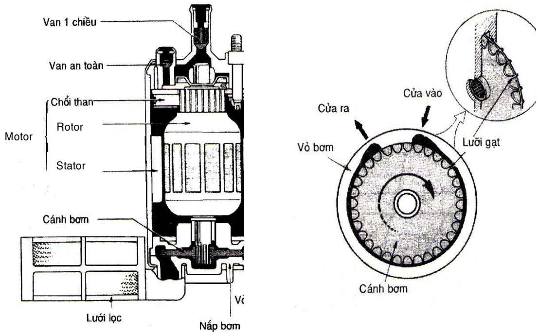
Hình 110: Bơm cánh quạt
