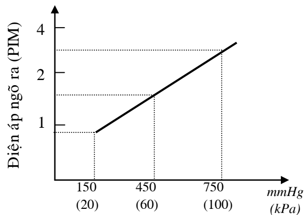
Hình 27: Đường đặc tuyến của MAP sensor
