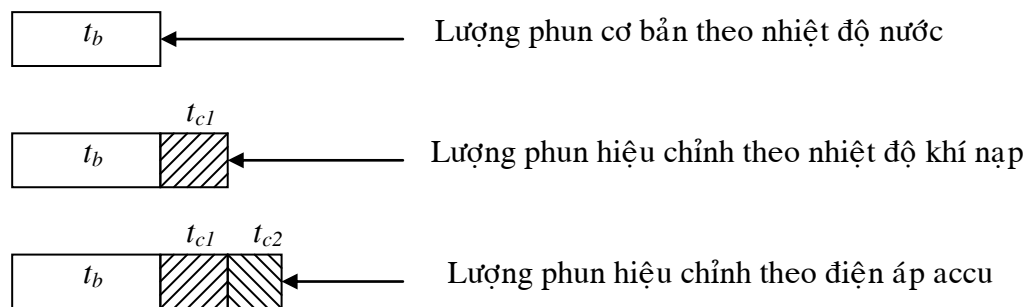
Hình 131: Điều khiển kim phun khi khởi động
