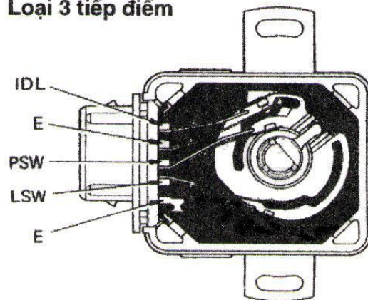
Hình 48: Cảm biến bướm ga có thêm công tắc cháy nghèo (LSW)
