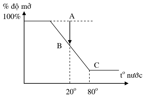
Hình 143: Điều khiển cầm chừng ở chế độ hâm nóng
