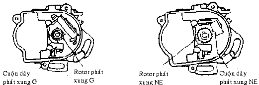
Hình 30: Sơ đồ bố trí cảm biến G và NE trên xe TOYOTA
