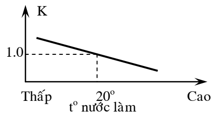
Hình 132: Đặc tính hiệu chỉnh bởi nhiệt độ khí nạp
