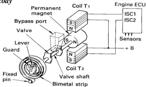
Hình 154: Cấu tạo van điều khiển cam chùng kiểu van xoay
