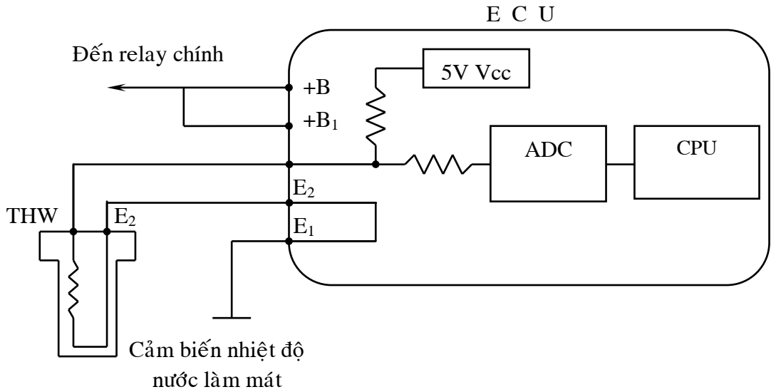
Hình 51: Mạch điện cảm biến nước làm mát
