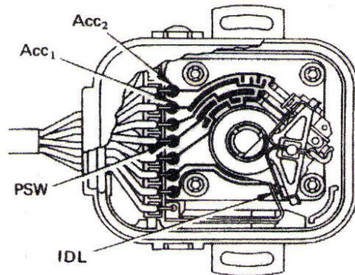
Hình 47: Cảm biến có công tắc ACC1 và ACC2
