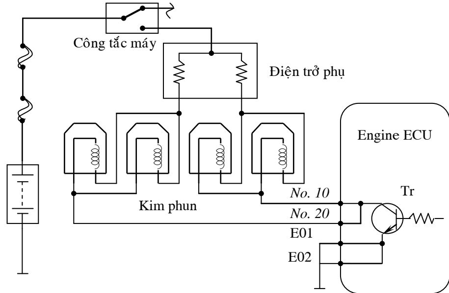
Hình 124: Mạch điện kim phun có điện trở thấp
