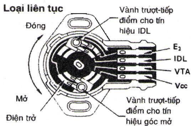
Hình 44: Cảm biến cánh bướm ga loại biến trở
