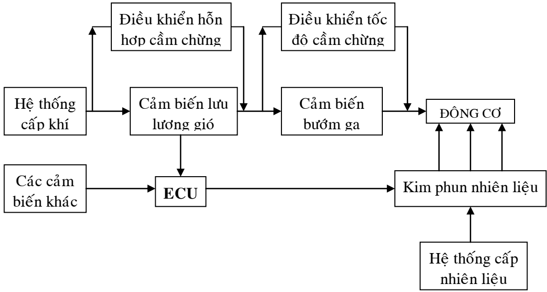
Hình 3: Sơ đồ các khối chức năng của hệ thống điều khiển phun xăng
