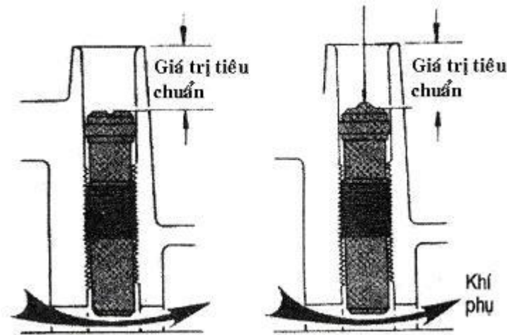
Hình 6: Vít chỉnh hỗn hợp cầm chừng
