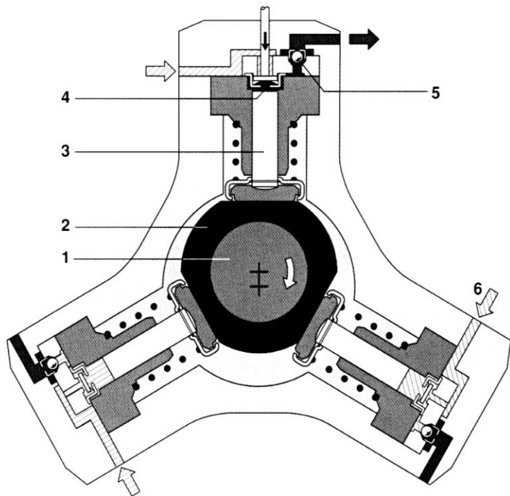
Hình 7.7. Bơm cao áp
