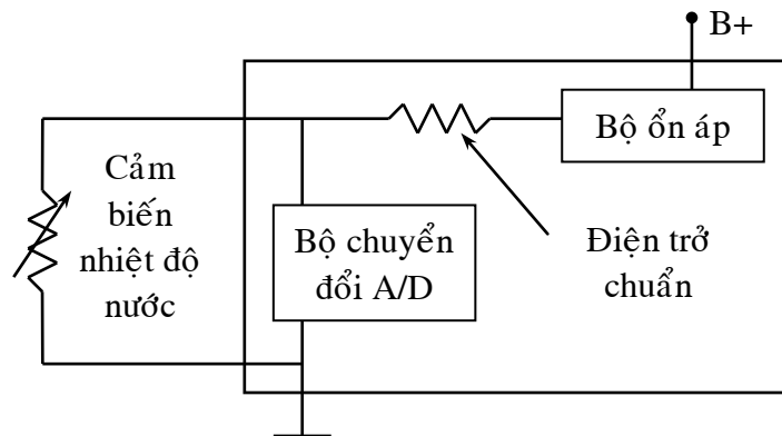
Hình 49: Mạch điện của cảm biến nhiệt độ nước làm mát
