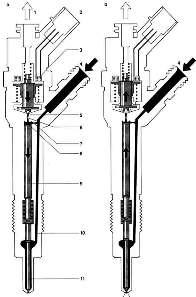
Hình 7.10: Cấu tạo kim phun
