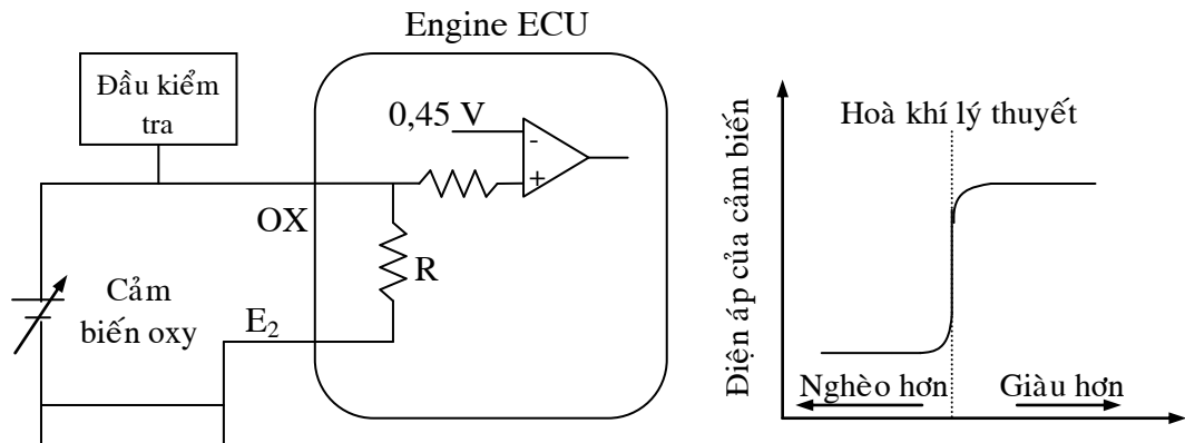
Hình 57: Mạch điện của cảm biến oxy loại zirconium
