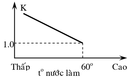
Hình 133: Sự hiệu chỉnh làm giàu sau khi khởi động
