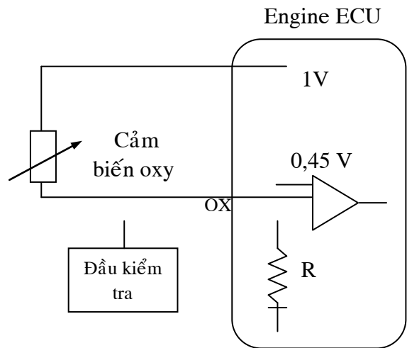
Hình 59: Mạch điện của cảm biến oxy loại titania
