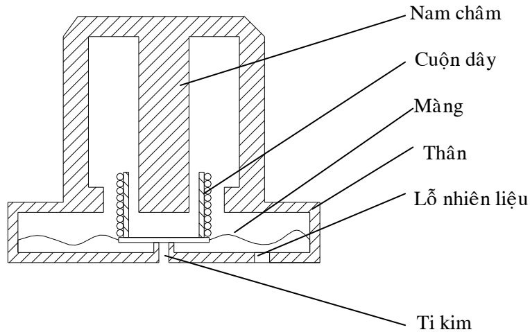
Hình 112: Biện pháp tăng độ chính xác trong hoạt động của kim phun
