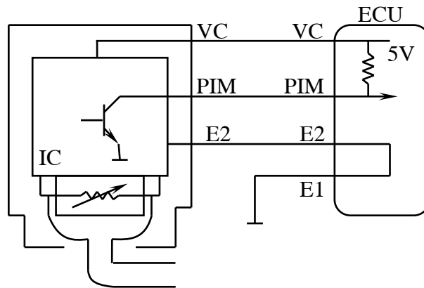
Hình 26: Mạch điện cảm biến áp suất đường ống nạp
