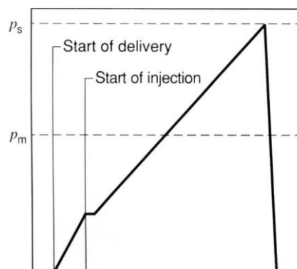
Hình 7.2: Đặc tính phun dầu thường
