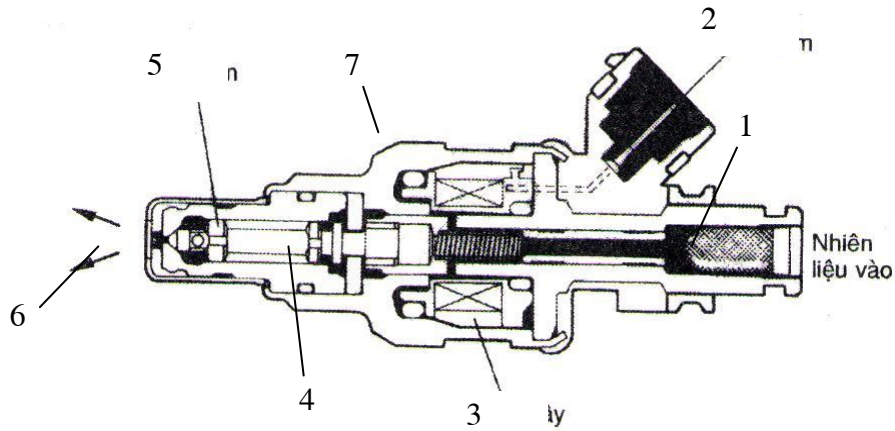
Hình 119: Kết cấu kim phun
