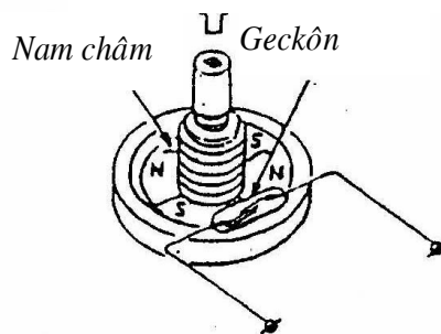
Hình 60: Cảm biến tốc độ xe
