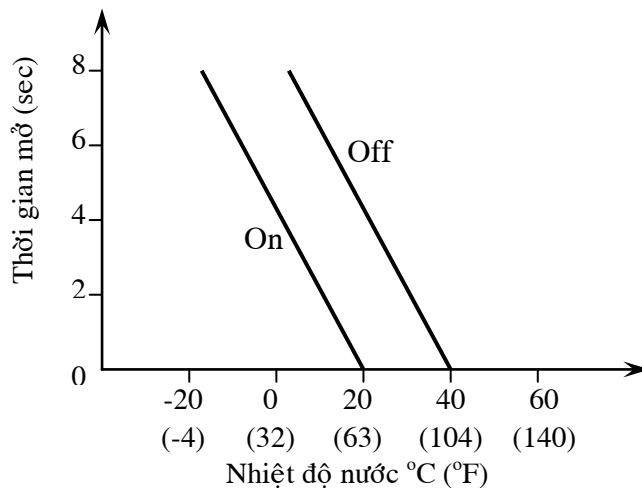
Hình 139 : Làm việc với kim phun khởi động lạnh
