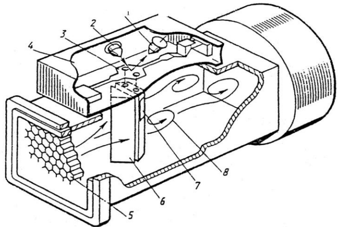
Hình 11: Bộ đo gió kiểu Karman quang
