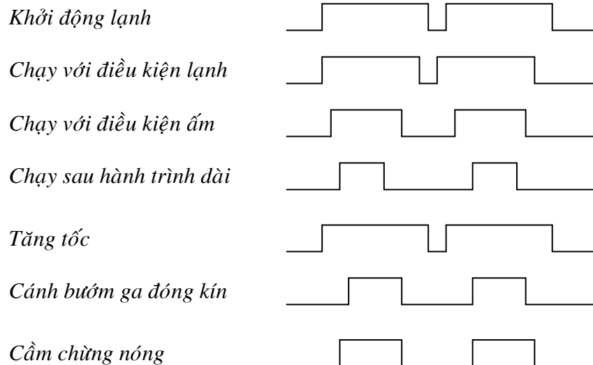
Hình 120: Xung điều khiển kim phun ứng với từng chế độ làm việc của động cơ
