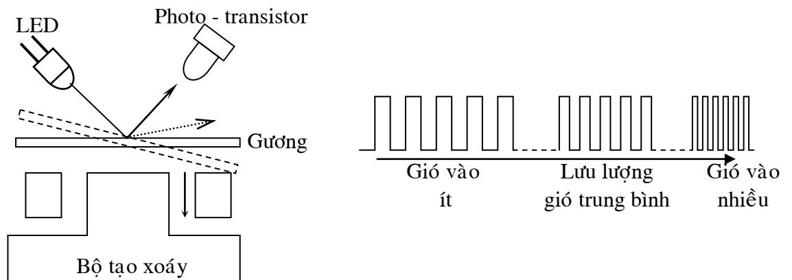
Hình 12: Cấu tạo và dạng xung loại Karman
