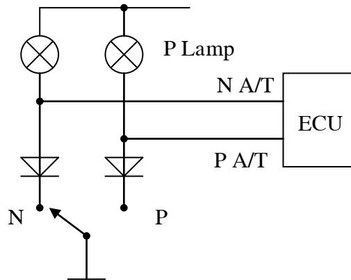
Hình 146: Tín hiệu từ hộp số tự động
