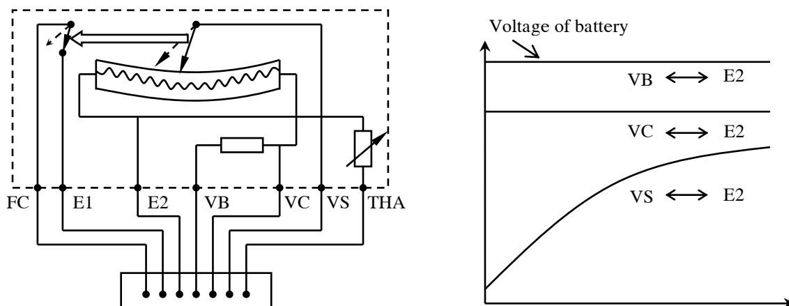
Hình 9: Mạch điện và đường đặc tuyến cảm biến đo gió loại điện áp tăng
