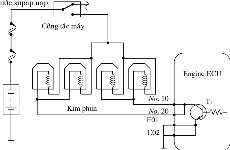
Hình 113: Mạch điện điều khiển kim phun bằng áp.
