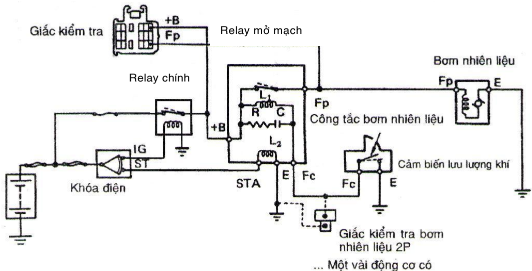
Hình 113: Mạch điện điều khiển bơm xăng không qua ECU
