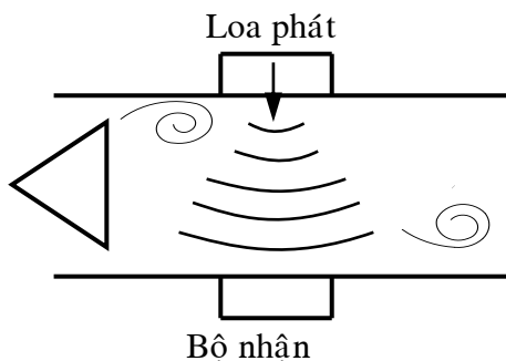
Hình 17: Dòng khí xoáy cùng chiều sóng siêu âm
