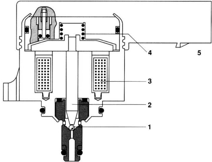
Hình 7.8: Cấu tạo van điều áp
