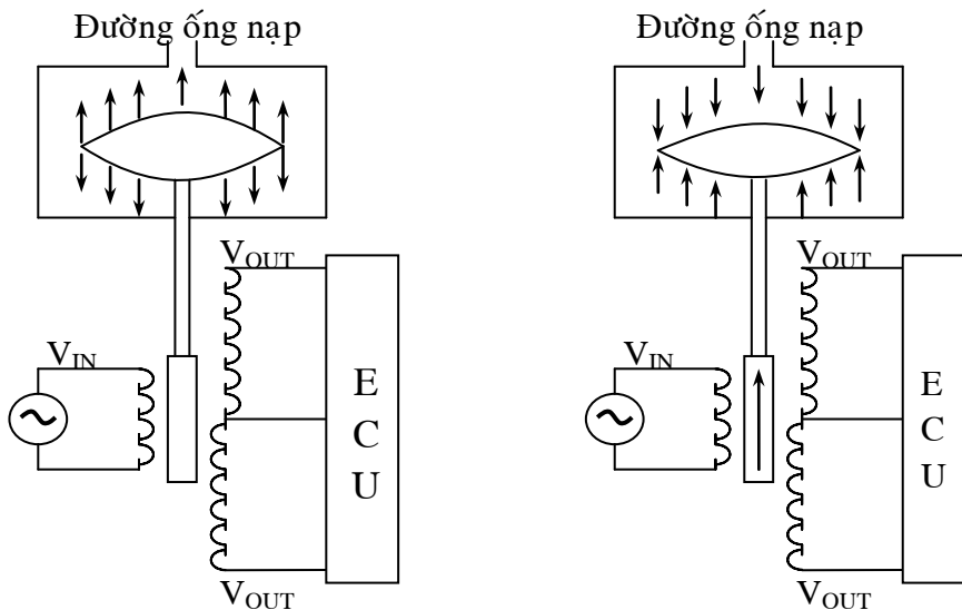
Hình 29: Sơ đồ nguyên lý MAP sensor loại sai lệch từ tuyến tính
