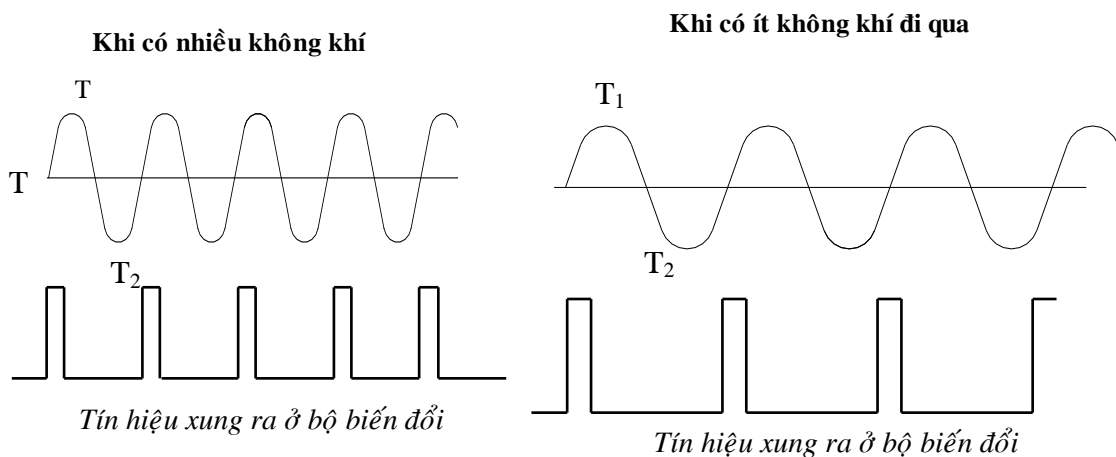
Hình 19: Xung ra của bộ đo gió Karman siêu âm thay đổi theo lưu lượng khí nạp
