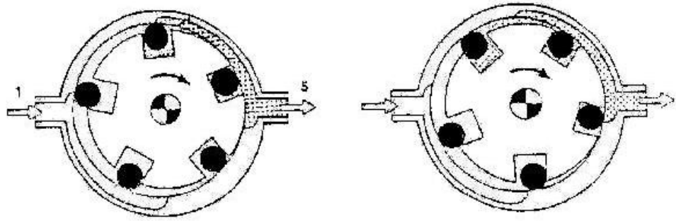
Hình 112 : Nguyên lý hoạt động của bơm con lăn
