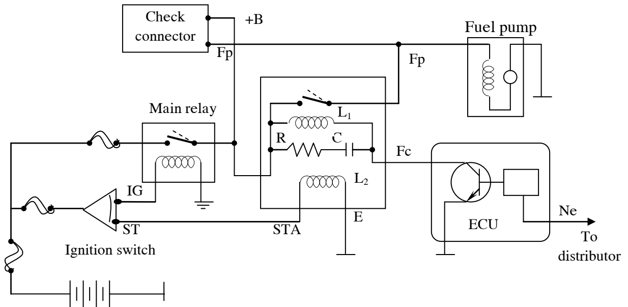
Hình 114: Mạch điện điều khiển bơm xăng có ECU điều khiển
