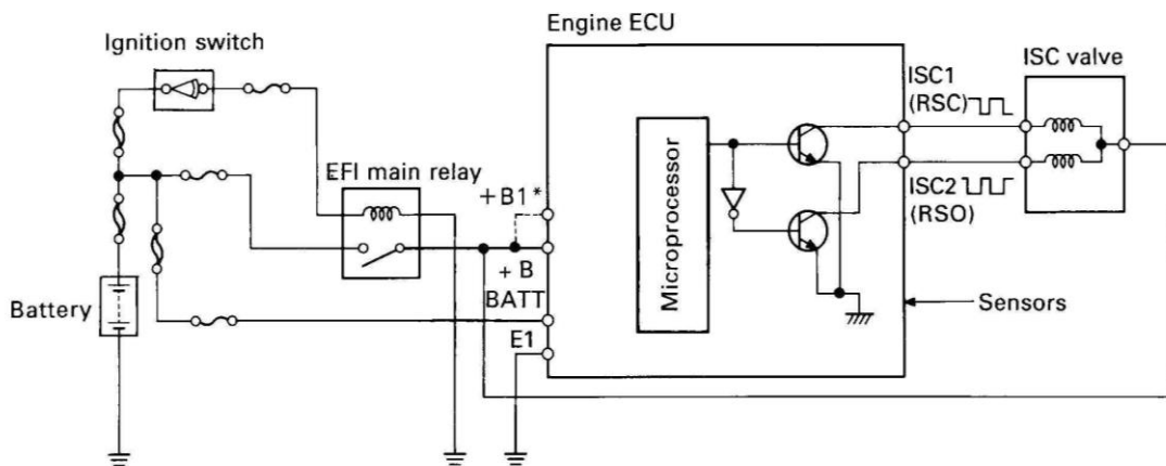
Hình 155: Mạch điện điều khiển cầm chừng dùng van xoay
