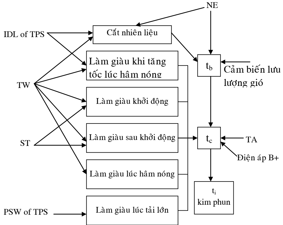
Hình 130: Điều khiển thời gian phun nhiên liệu
