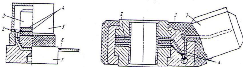
Hình 62: Cấu tạo cảm biến kích nổ 1. Đáy cảm biến; 2. Tinh thể thạch anh; 3. Khối lượng quán tính; 5. Nắp; 6. Dây đàn; 7. Đầu cảm biến
