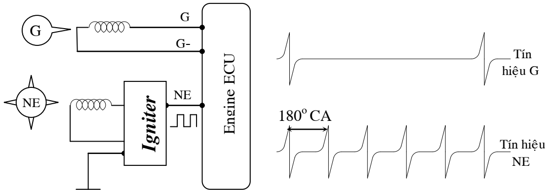
Hình 38: Sơ đồ và dạng xung của loại 4/4 kết hợp IC đánh lửa
