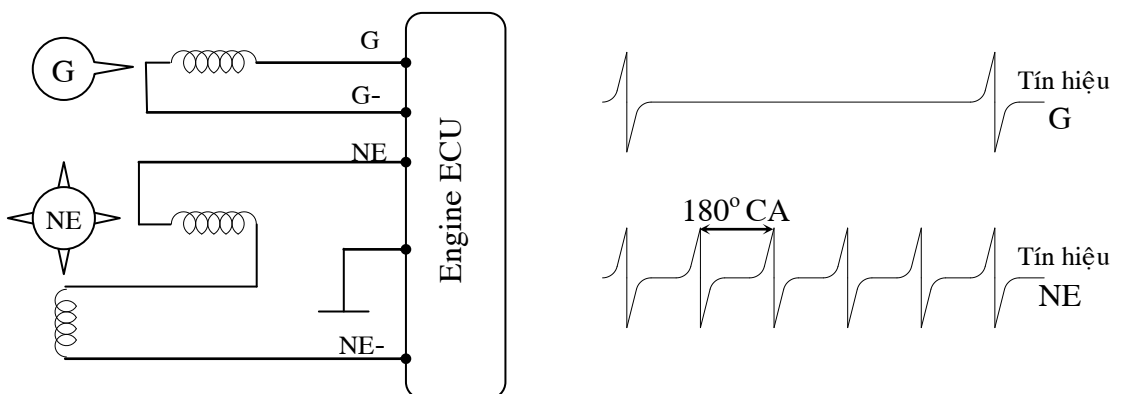
Hình 36: Sơ đồ và dạng xung loại 1/4
