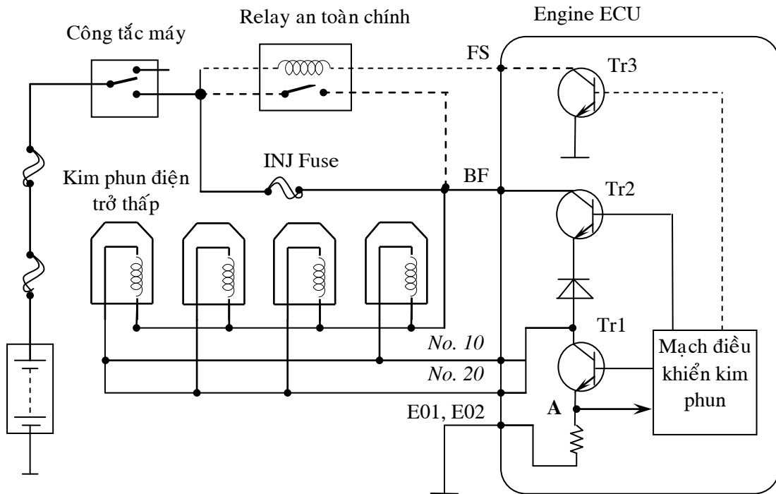
Hình 127: Mạch điện điều khiển kim phun bằng dòng
