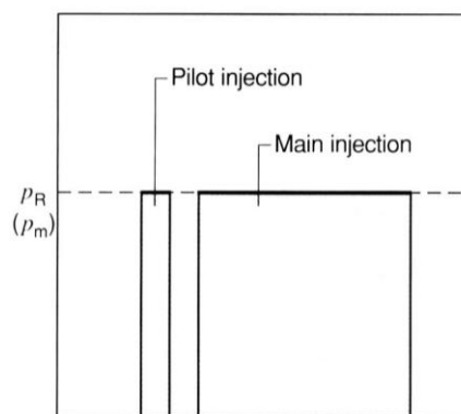
Hình 7.3: Đường đặc tính phun của hệ thống Common Rail.
