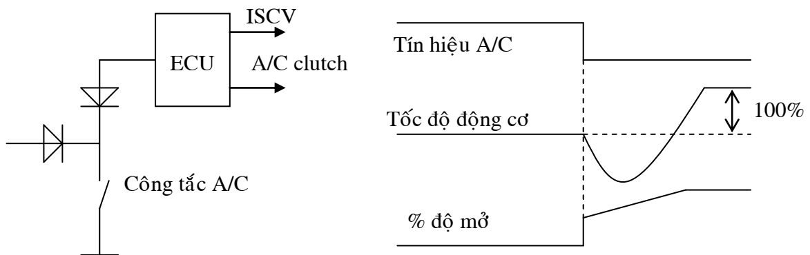
Hình 144: Chế độ máy lạnh
