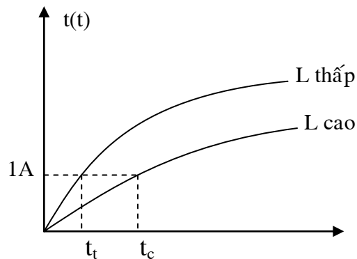
Hình 128: Đồ thị biểu thị sự ảnh hưởng của độ tự cảm L
