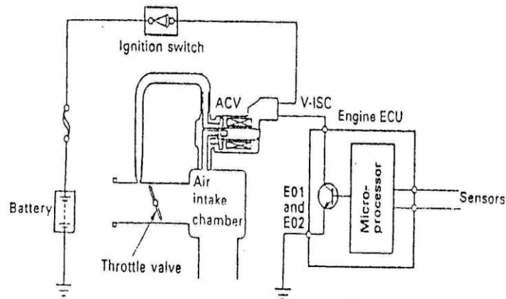
Hình 153: Mạch điện của van điều khiển cam chùng kiểu solenoid
