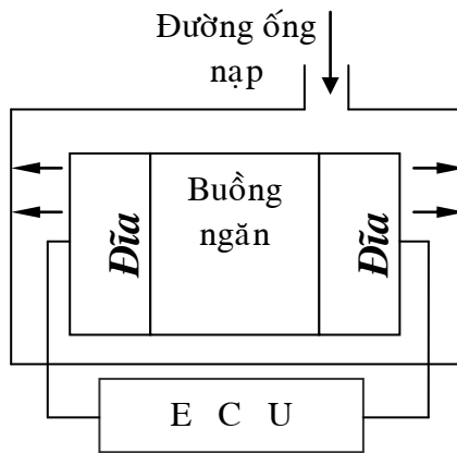
Hình 28: Sơ đồ cấu tạo cảm biến MAP loại điện dung
