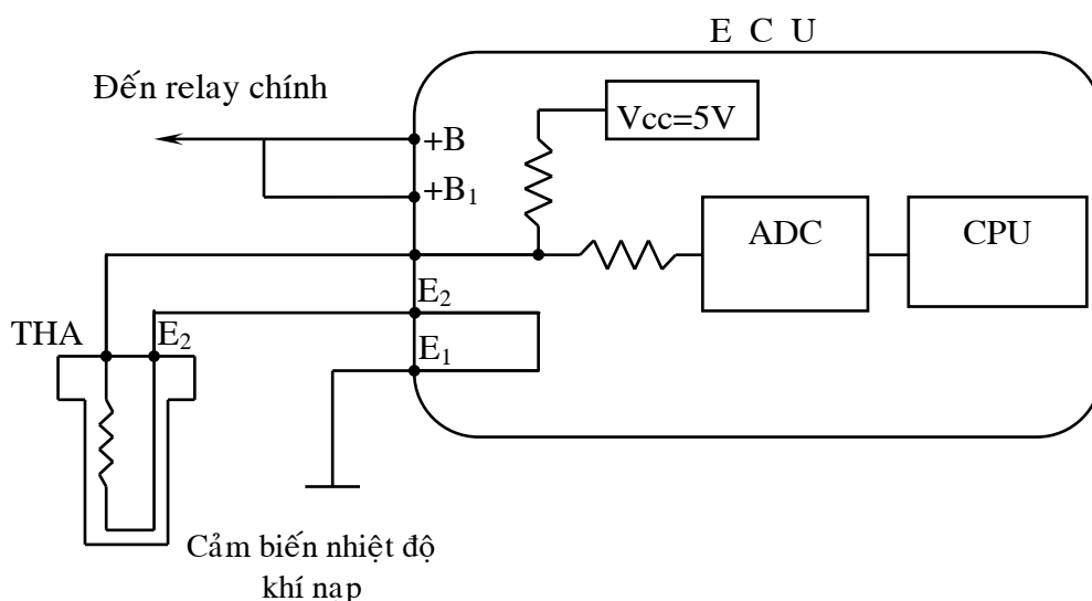
Hình 54: Mạch điện của cảm biến nhiệt độ khí nạp
