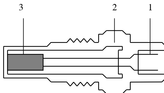
Hình 50: Cảm biến nhiệt độ nước làm mát
