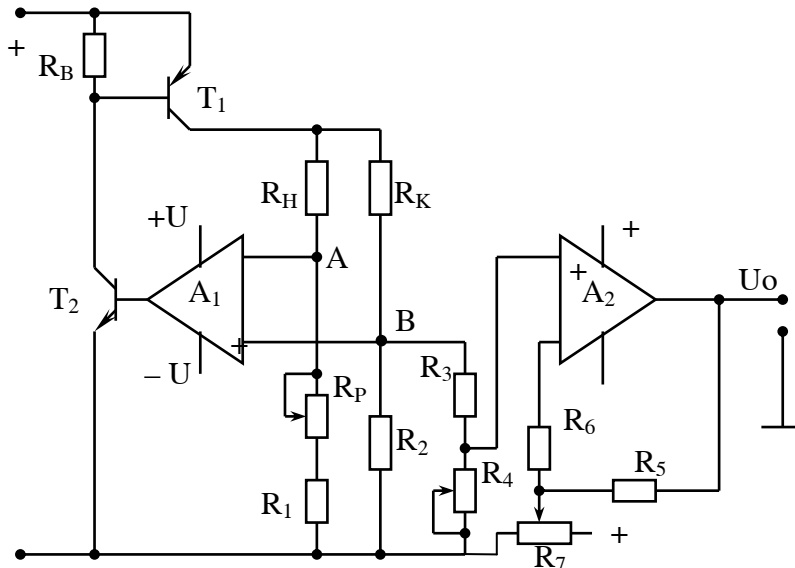
Hình 21: Mạch điện cảm biến đo gió kiểu dây nhiệt
